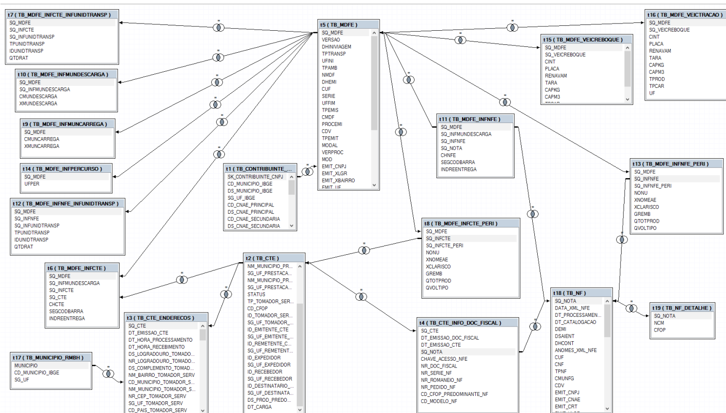
Figura 5 – Tabelas das bases de dados utilizadas na construção da matriz de cargas
